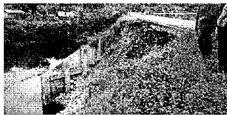
Colapso del relleno estribo del Puente Cabeno
